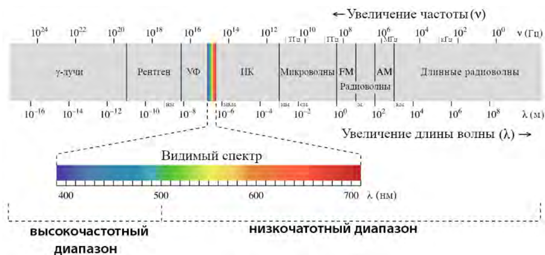
Рисунок 2. Электромагнитный спектр
